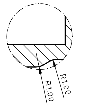
DETALLE E SIN ESCALA
