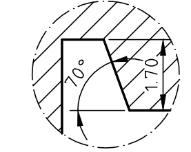
DETALLE A. SIN ESCALA
