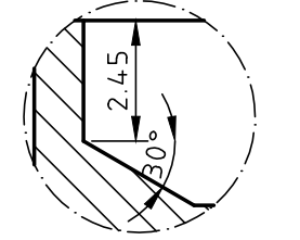
DETALLE D SIN ESCALA
